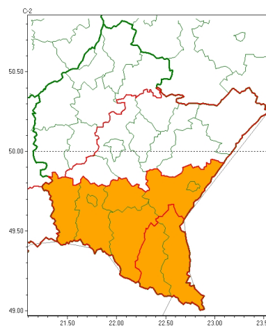
Opady marznące 2023-12-01 06:12
